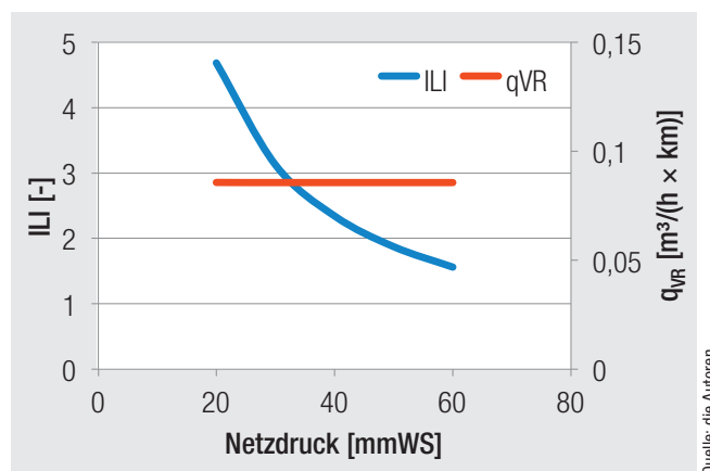
Abb. 2: Vergleich ILI und q_{VR} bei wechselndem Wasserdruck
